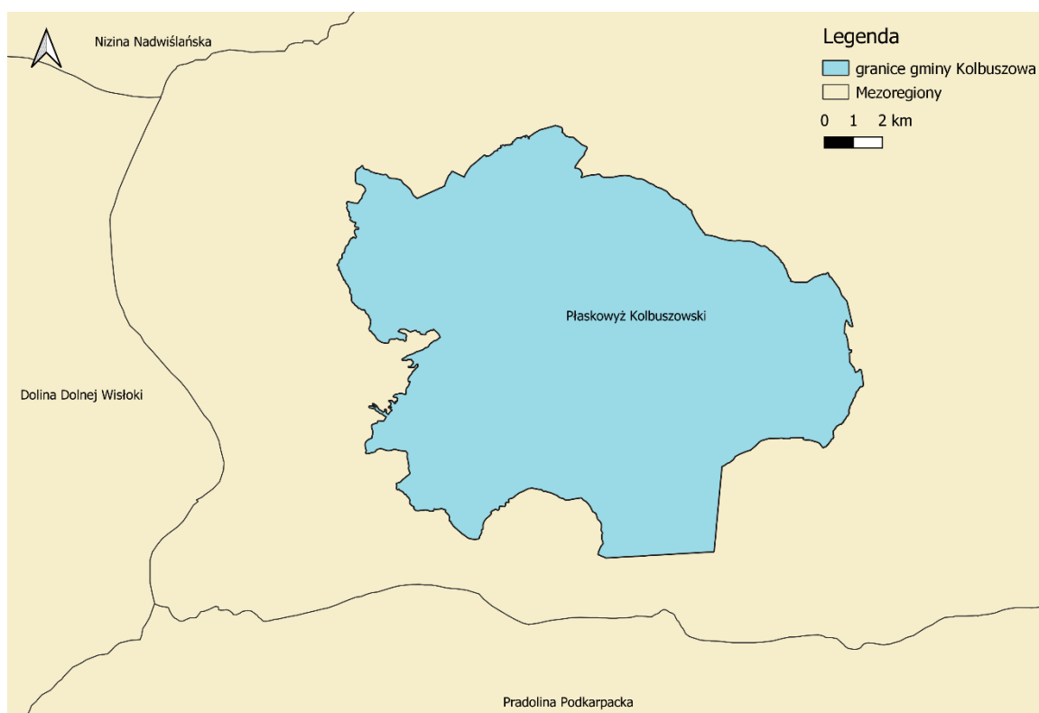
Rysunek 3. Położenie gminy Kolbuszowa na tle mezoregionów źródło: Centralna Baza Danych Geologicznych, opracowanie własne
